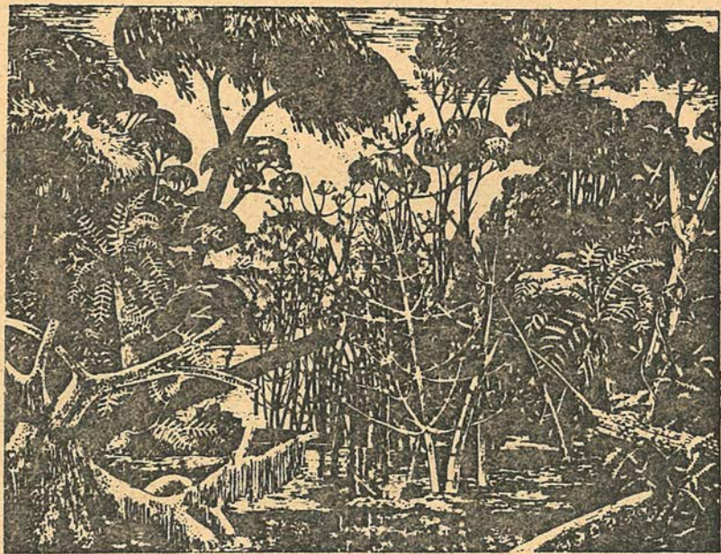
Обр. 4. Рослинність кам'яновугільного періоду.
