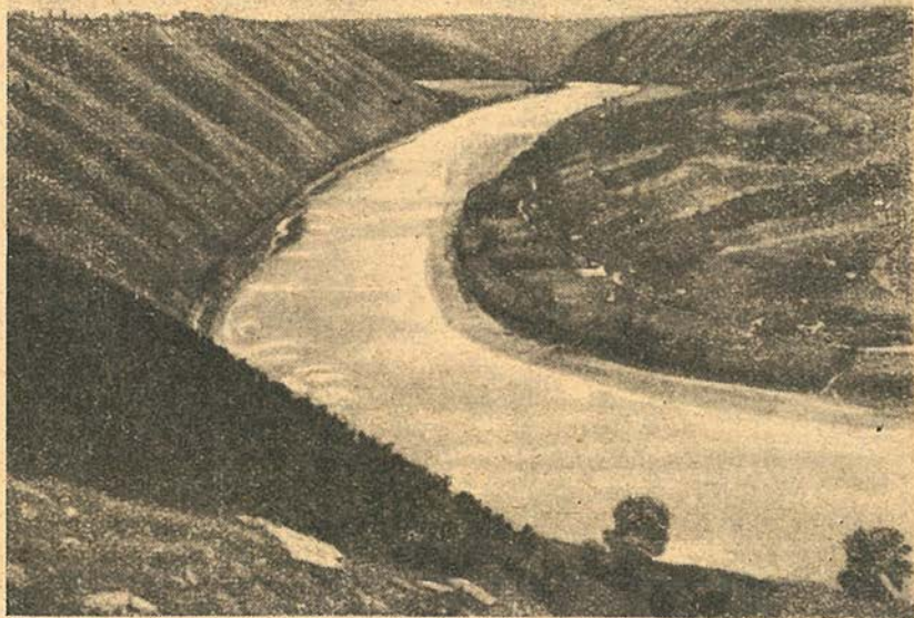
Обр. 25. Село Сокирчин в ярі Дністра у Галичині.
